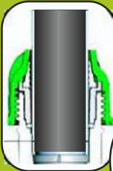
O-ring'in boru içine girdikten sonraki kilitli pozisyonu final, lock position of the o-ring with the pipe in its place.
