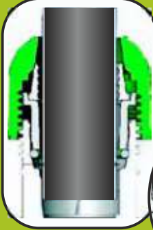
boru girişı sırasında O-ring'in gevşek hali Release position of the O-ring while the pipe is being inserted.
